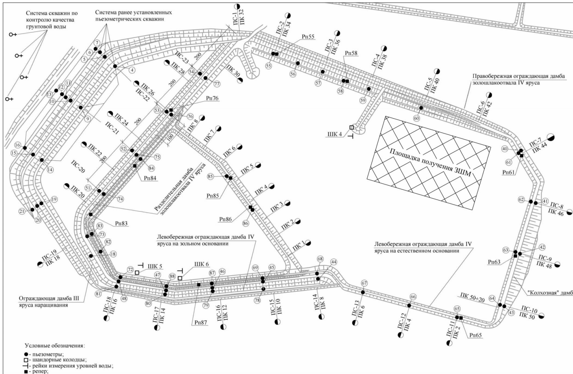
Рисунок 1 - План-схема золоотвала Беловской ГРЭС
