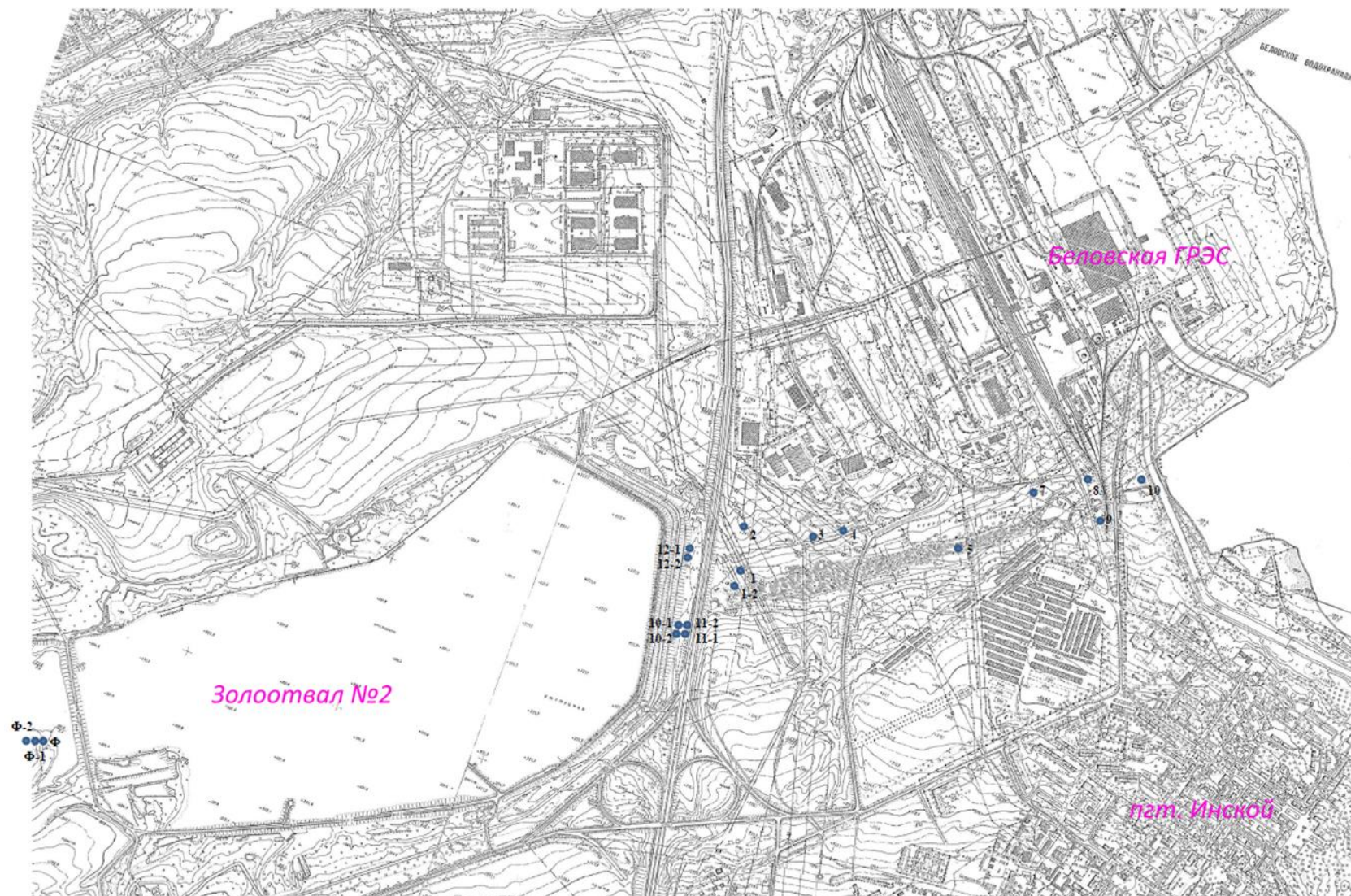
Рисунок 3 – Карта-схема расположения пьезометрических скважин на золотвале №2 Беловской ГРЭС ОАО «Кузбассэнерго»
